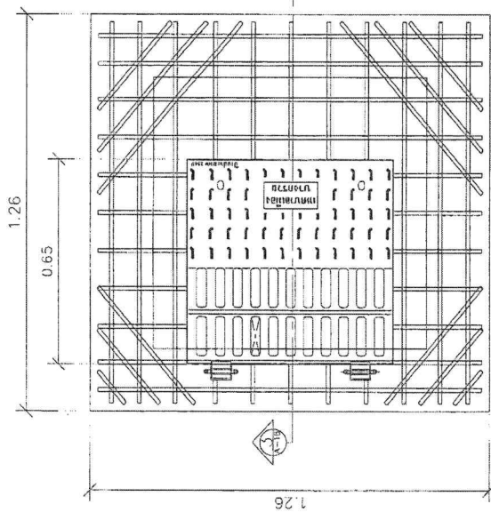
แปลนขยายเหล็กผ้าบอมบ์รังวิ มาตราส่วน 1:15
