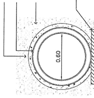
รูปตัดรอยต่อท่อระบายน้ำตามขวาง มาตราส่วน 1 : 20
