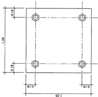
แบบแปลนสำเนา บอพักหอระบายน มาตราส่วน 1 : 25
