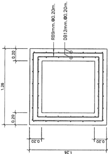
แบบขยายเหล็กเสริม บอพักอะระบายน้ำ มาตราส่วน 1 : 25
